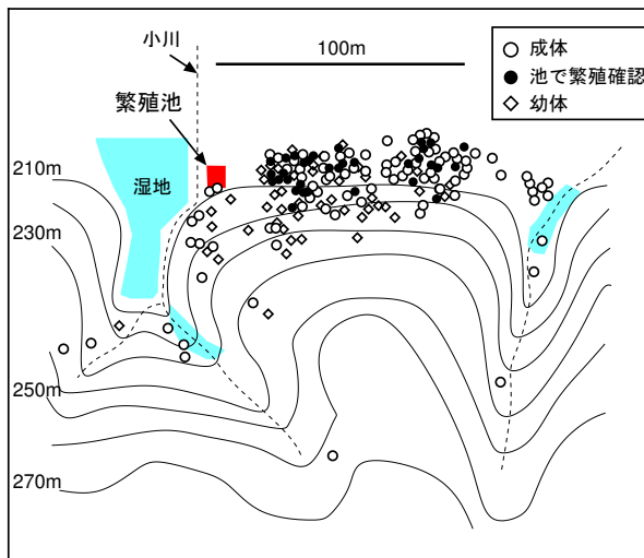
図 2.12: トウキョウサンショウウオの非繁殖期の分布。文献 [28] より。
