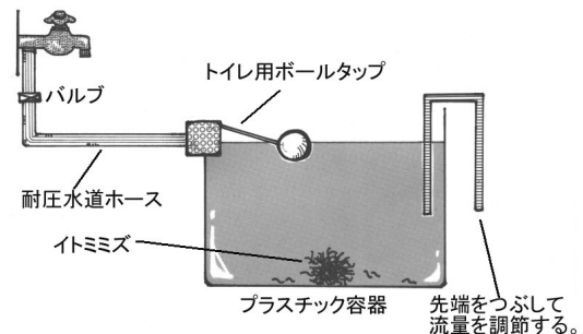
図 B.5: イトミミズ飼育装置の一例。
